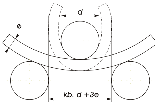
A hajlítási próba vázolata
