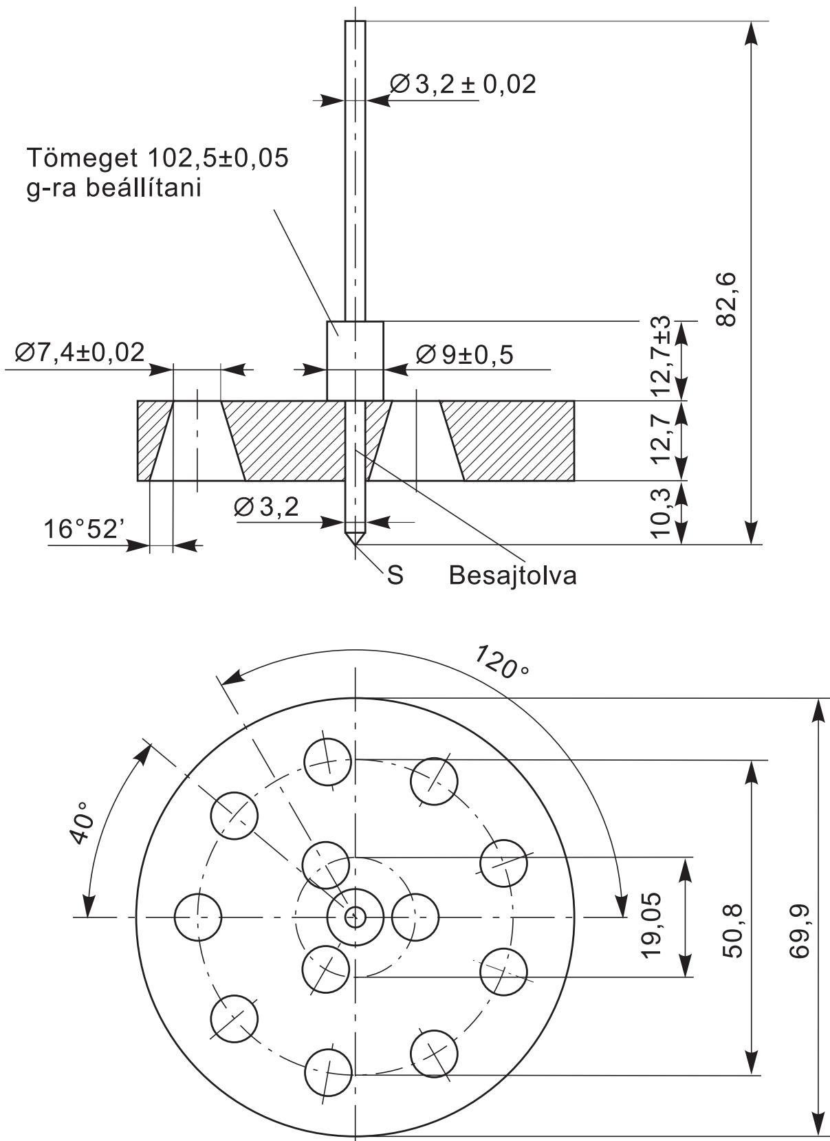
4. ábra: Penetrométer
