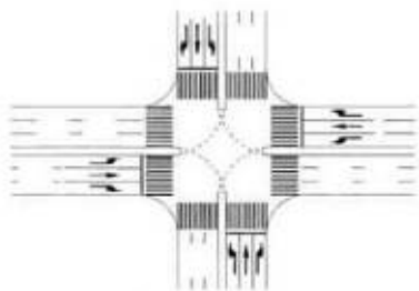
Marcaj de ghidare în intersecție
